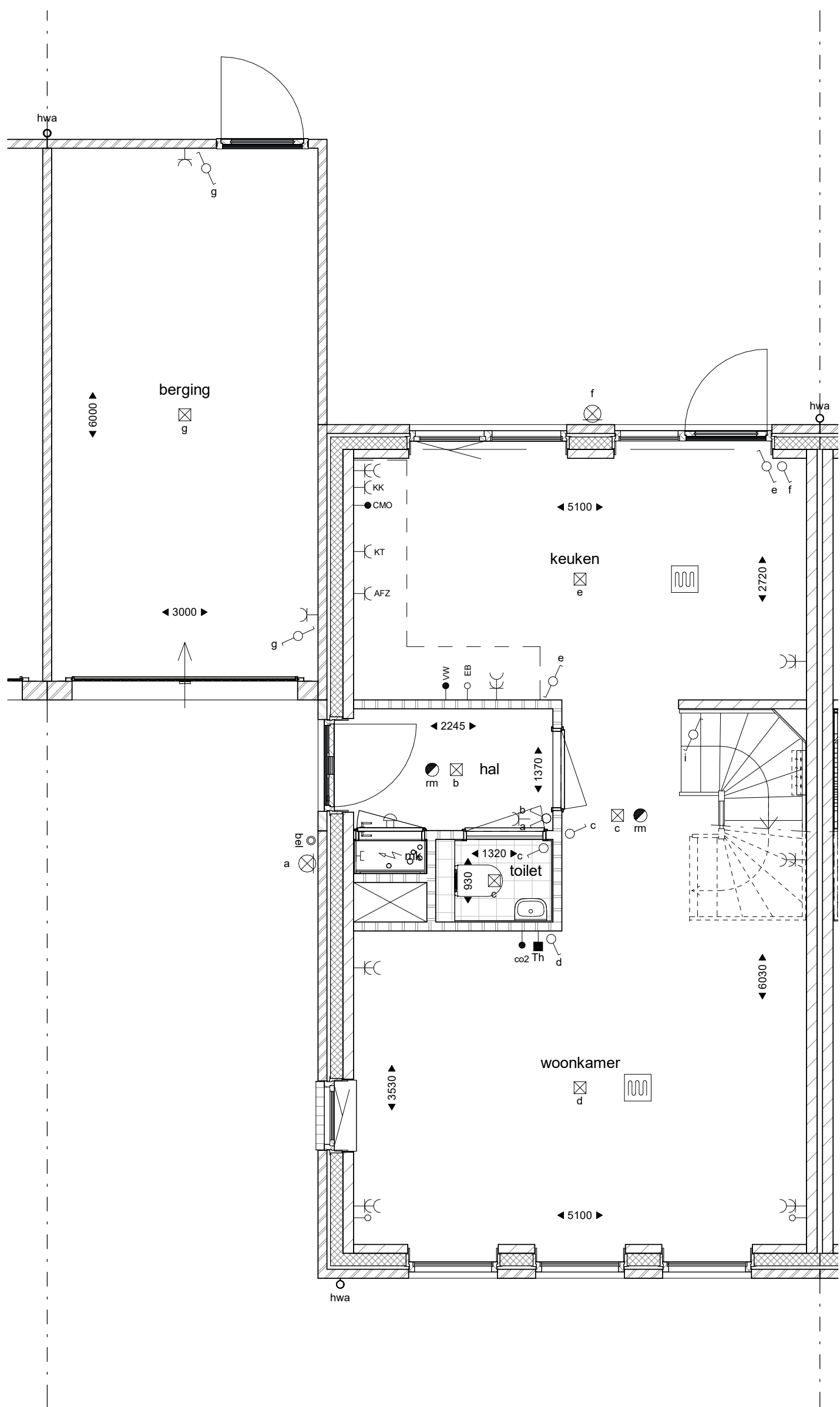
begane grond 1 : 50
