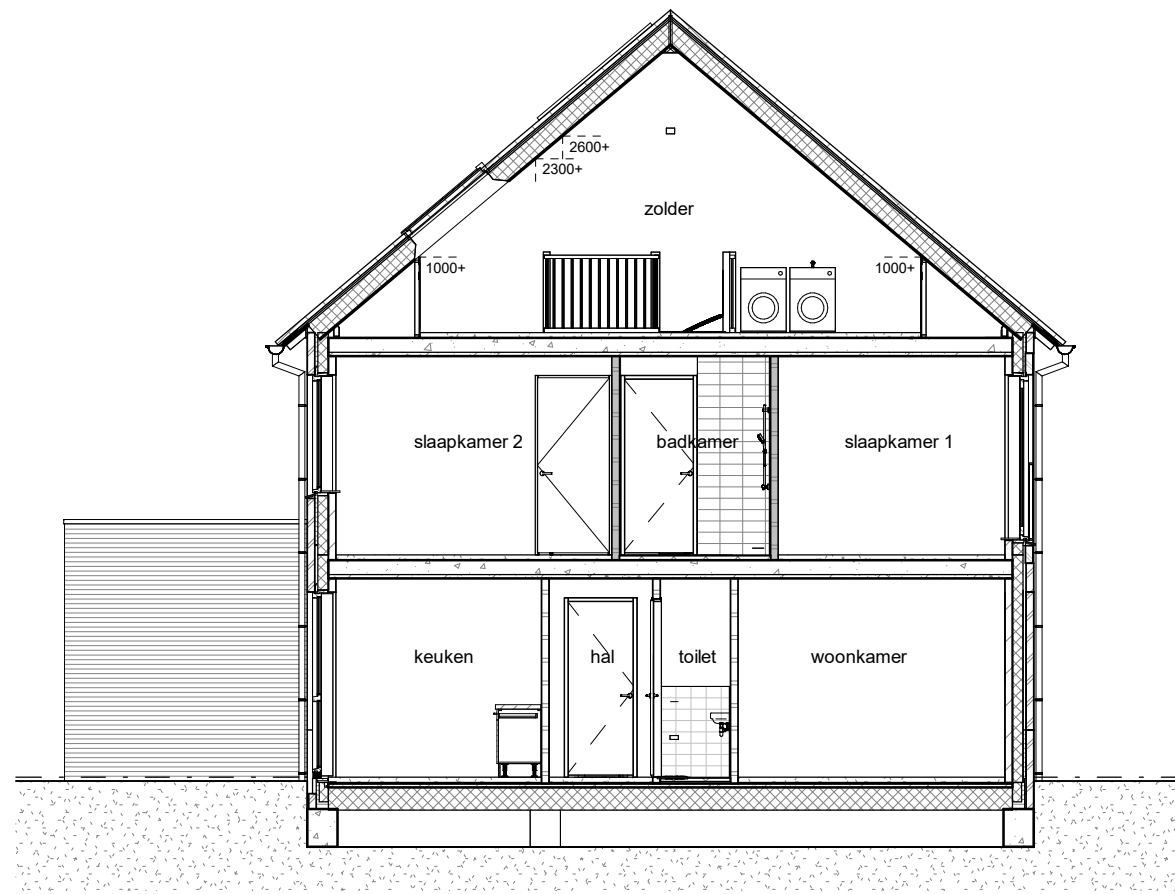
doorsnede 1 : 100
