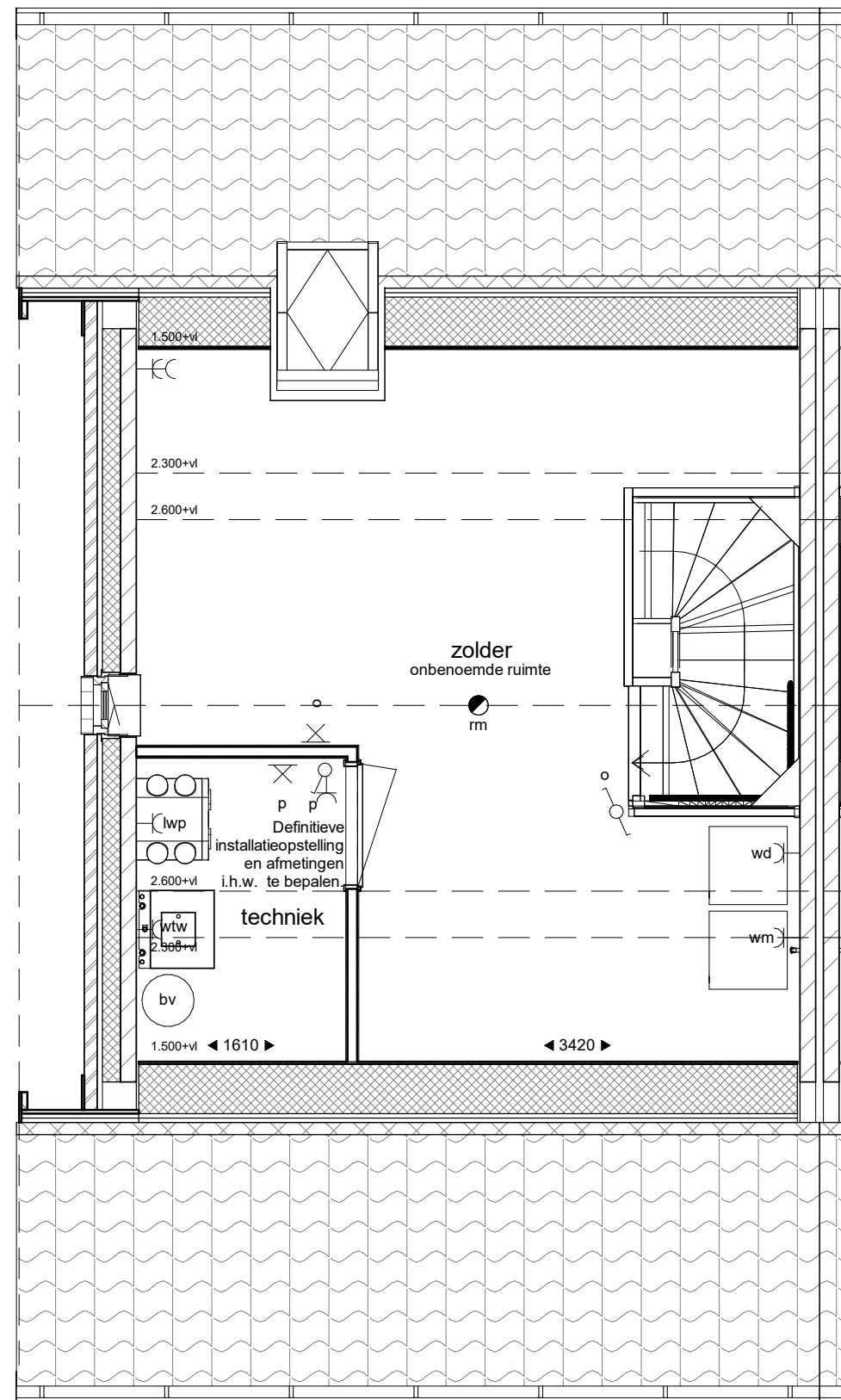
tweede verdieping 1 : 50
