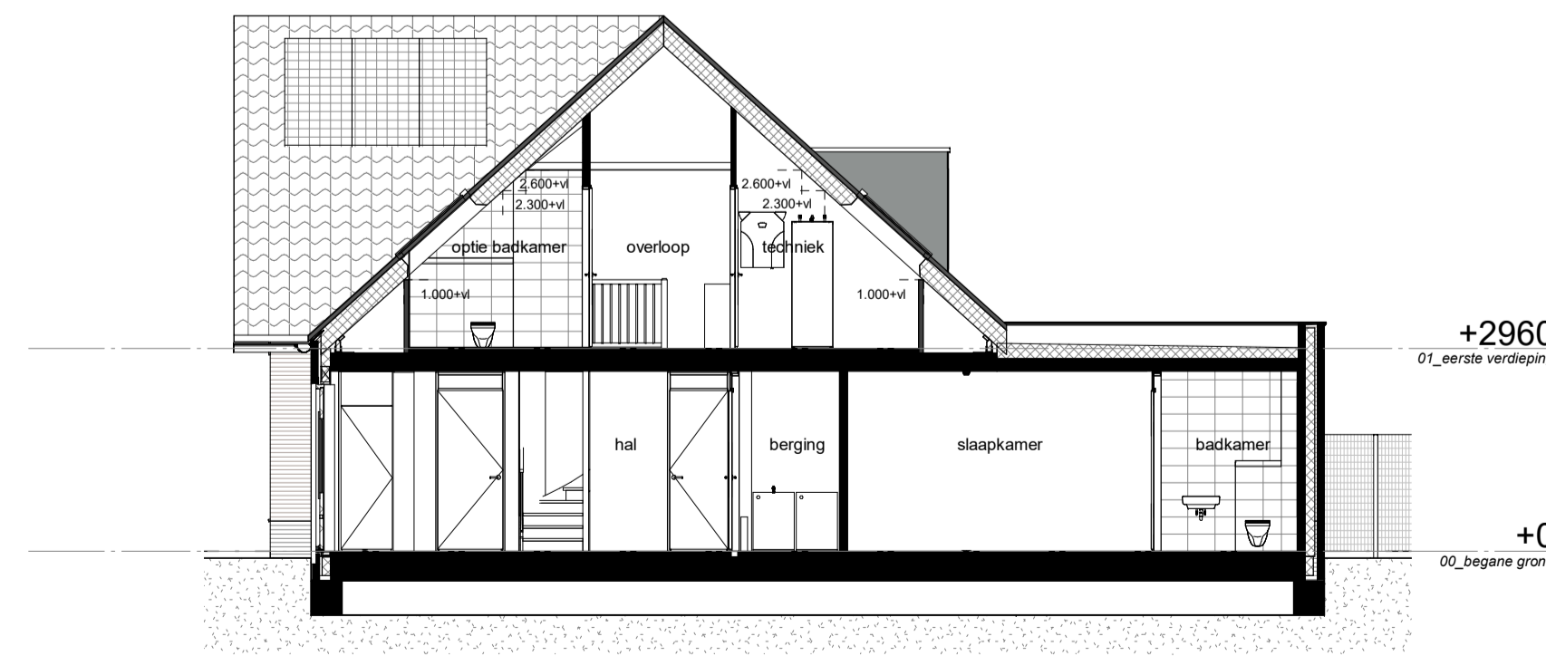
doorsnede 1 : 100
