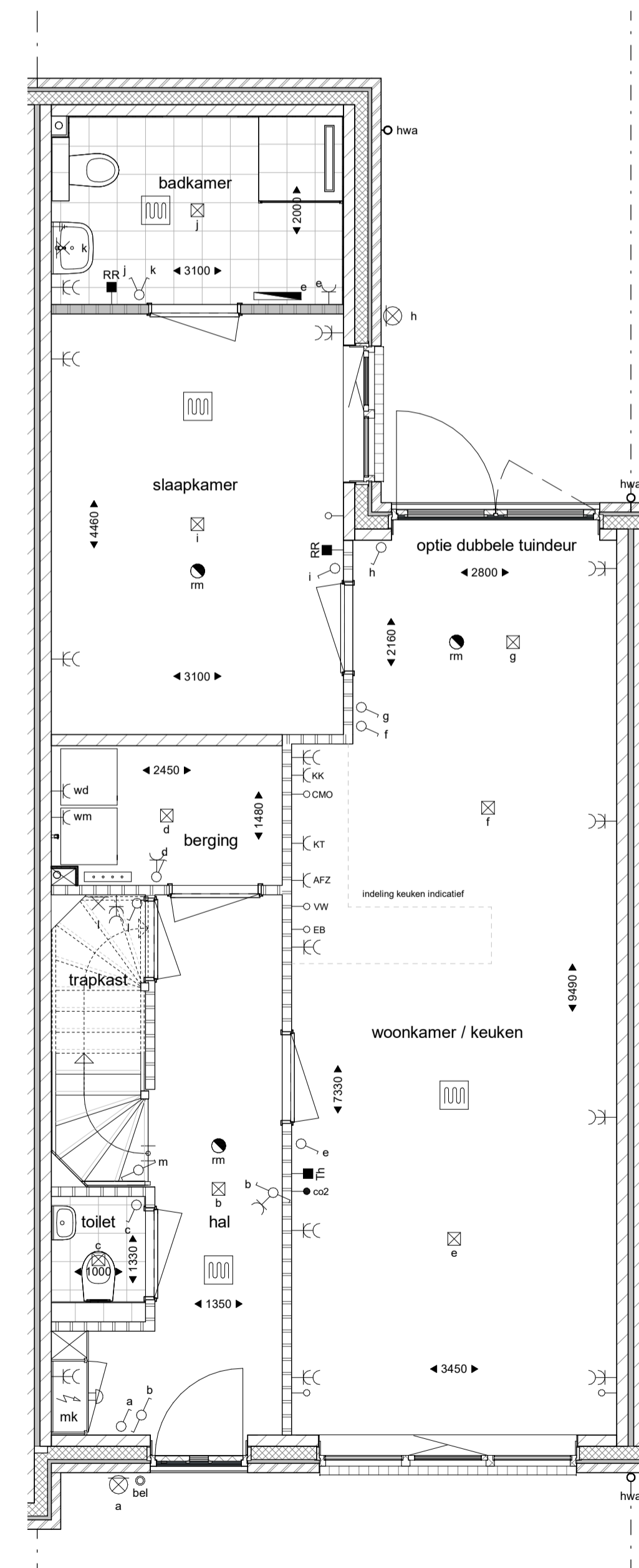
begane grond 1 : 50
