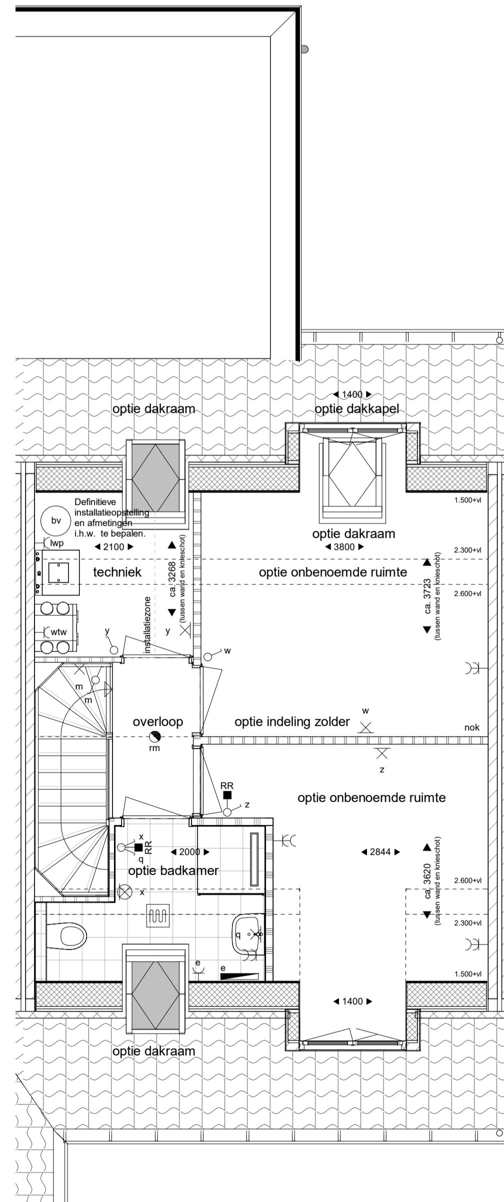
eerste verdieping 1 : 50
